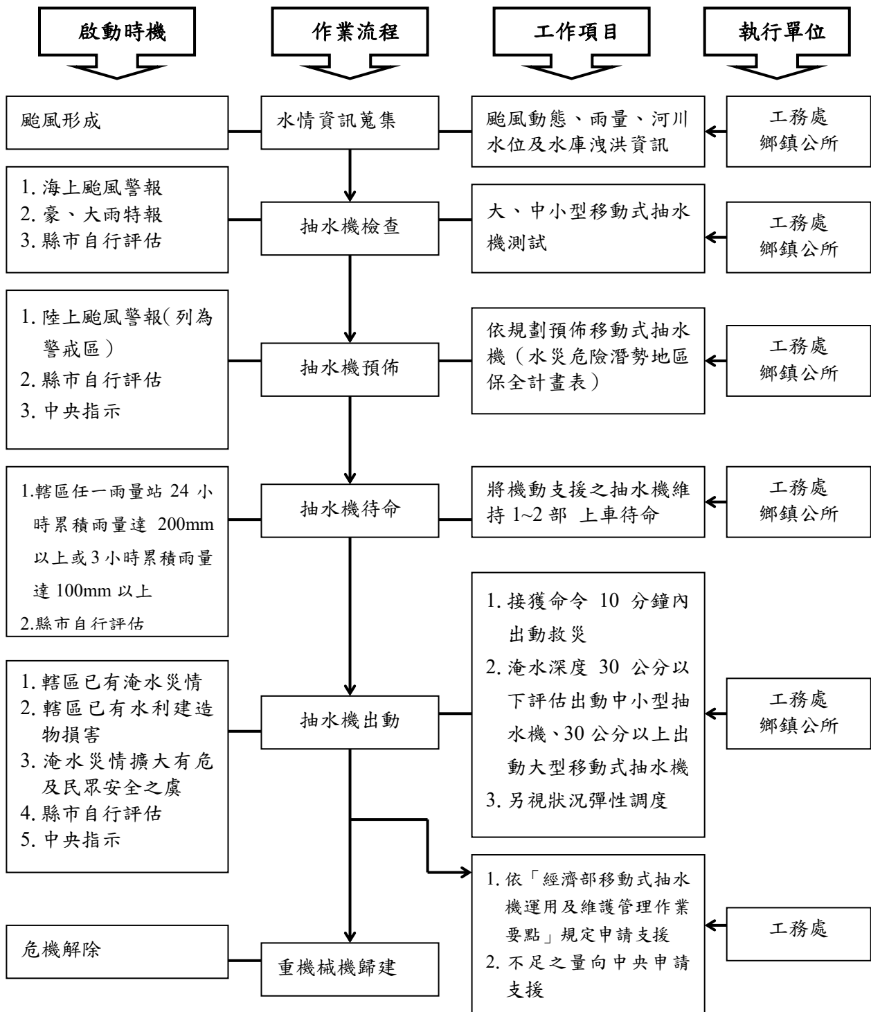
圖 3-3 移動式抽水機運用流程圖
